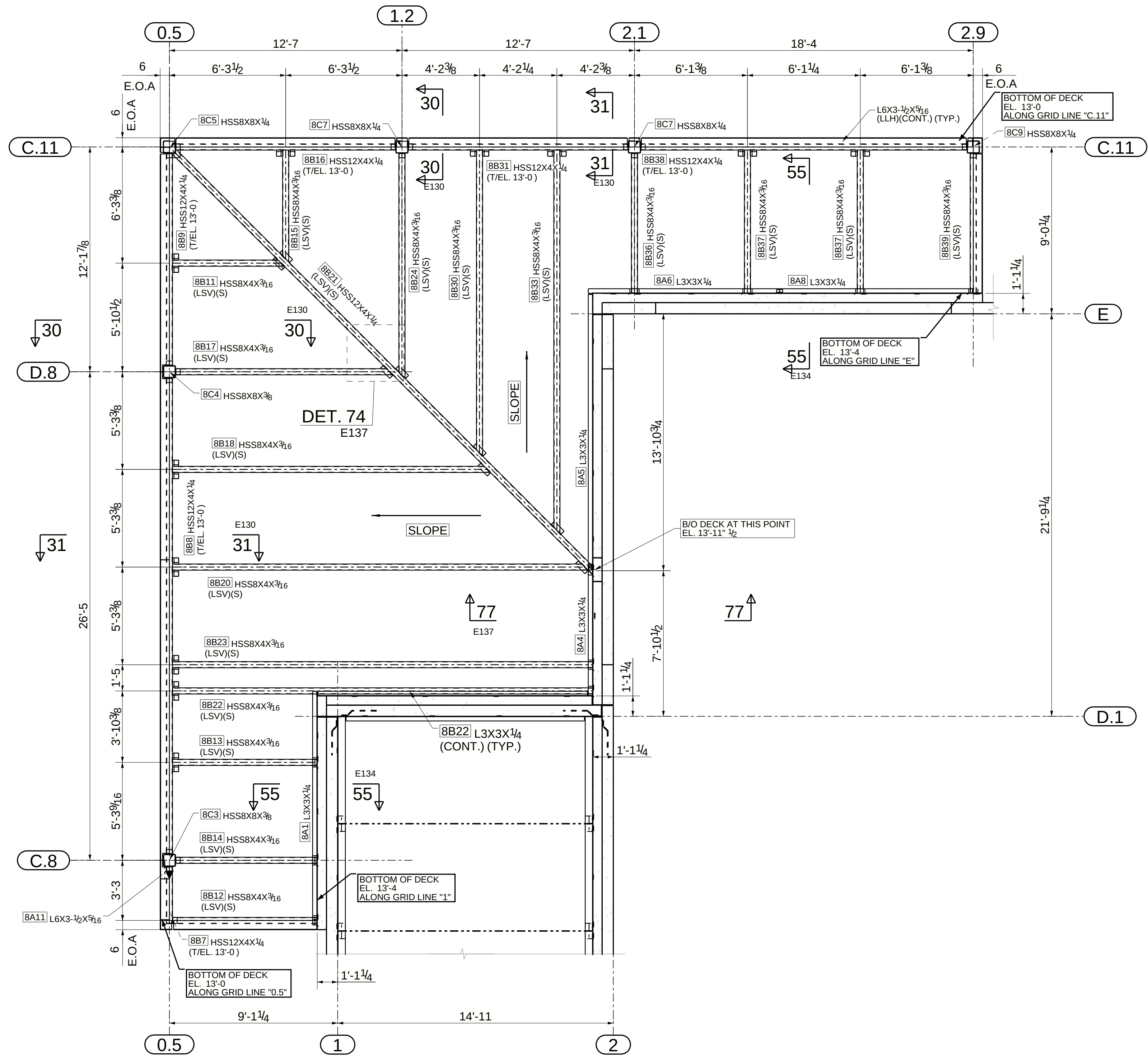
DETAIL V E101 CANOPY FRAMING PLAN
