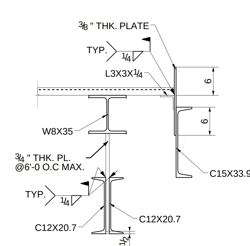
SECTION Q1 - Q1
